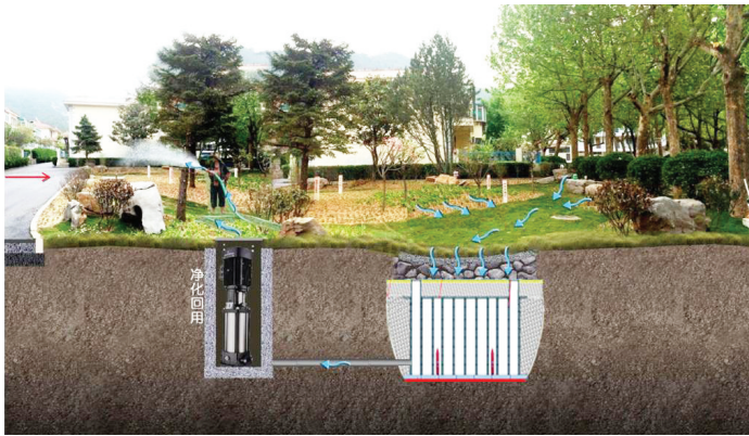
雨水收集利用示意图
